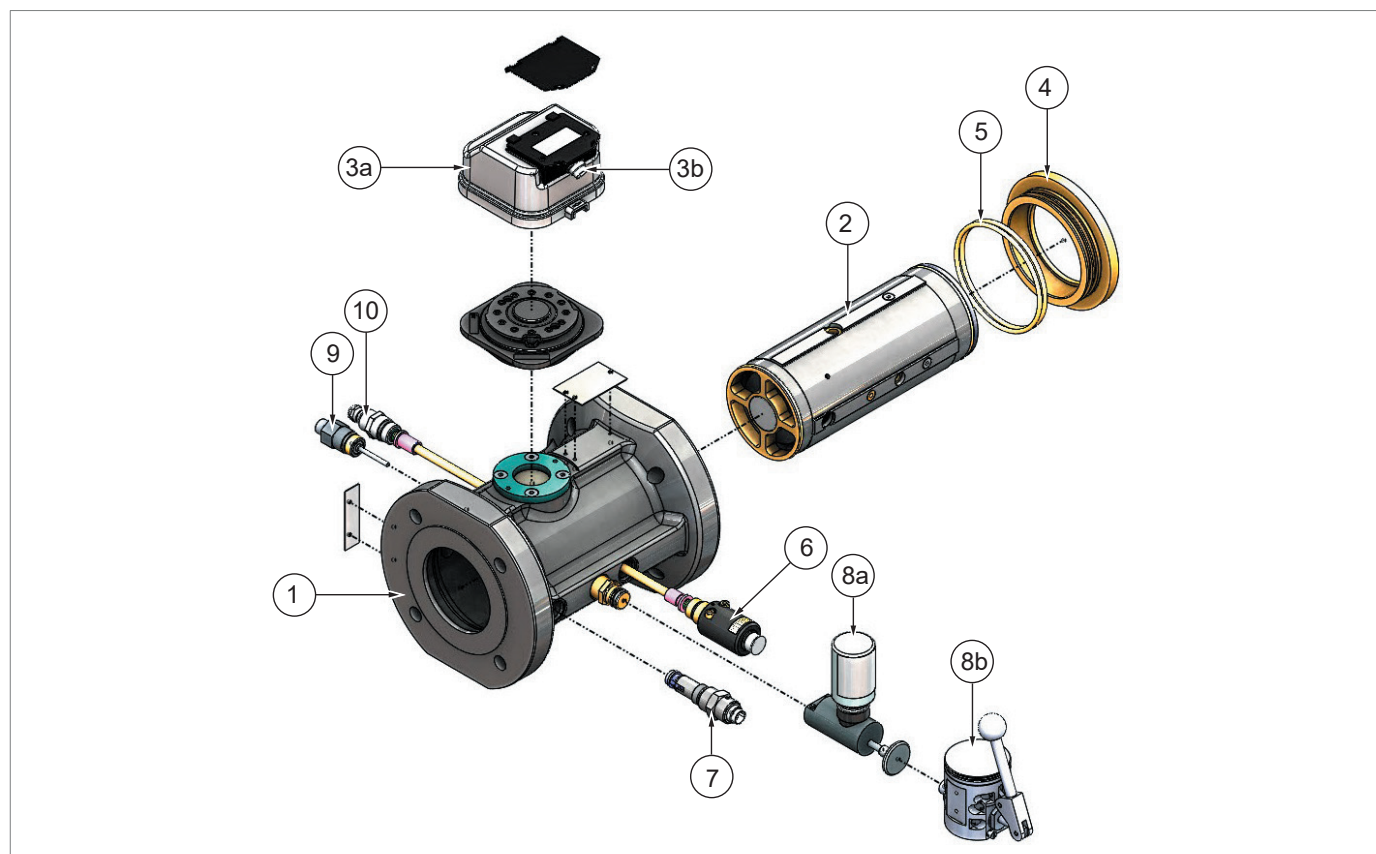
Fig. 4.2. Description générale iM-TM
