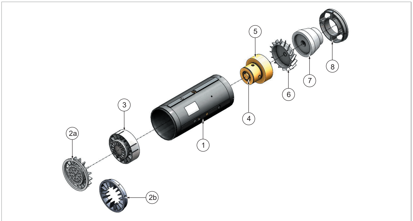
Fig. 4.3. Groupe cartouche de mesure
