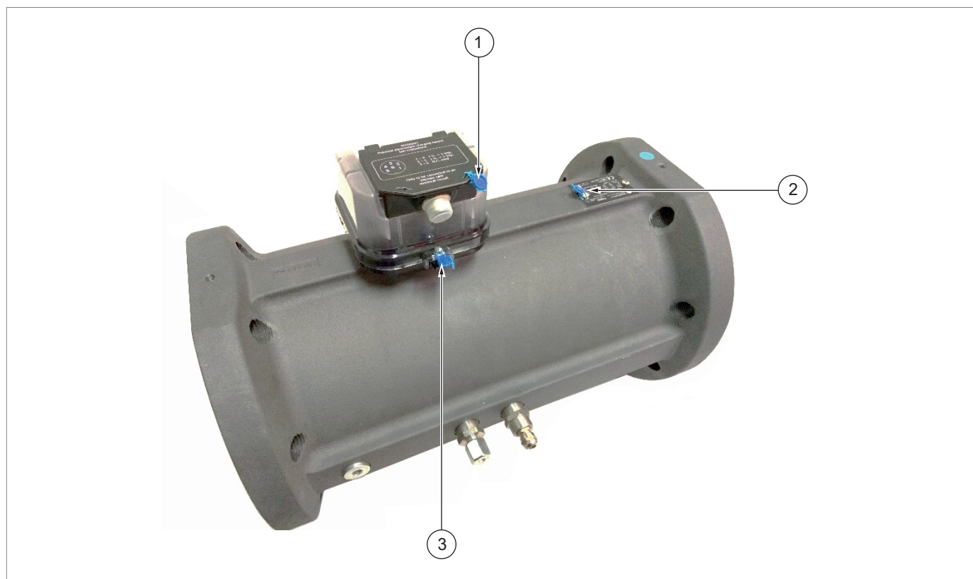
Fig. 4.5. Emplacement des scellés métrologiques
