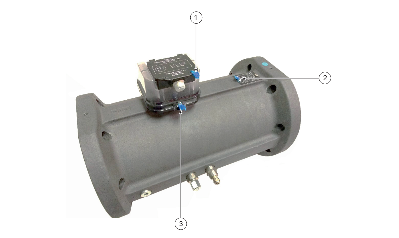
Fig. 4.5. Colocación de precintos metrológicos
