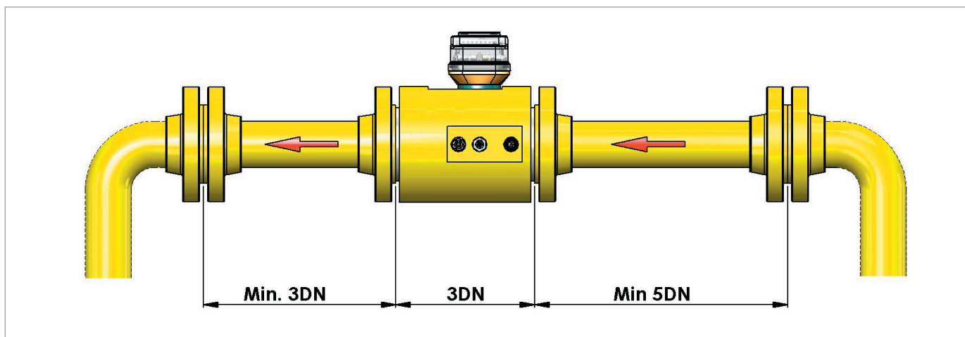
Fig. 6.11. Instalación recomendada iM-TM
