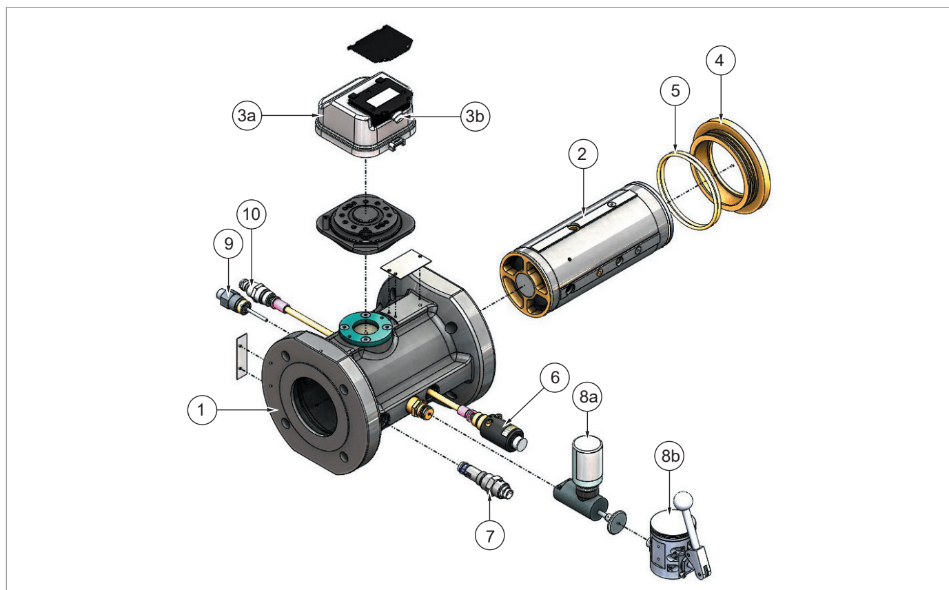
Fig. 4.2. Descripción general iM-TM
