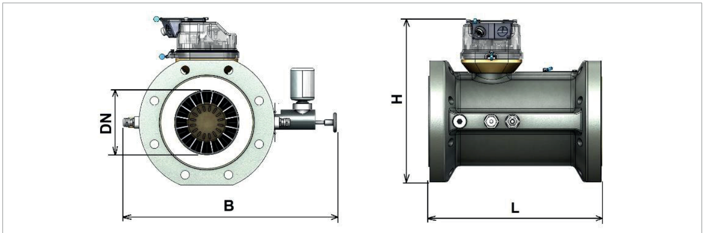
Fig. 5.7. Características físicas iM-TM cuerpo de aluminio
