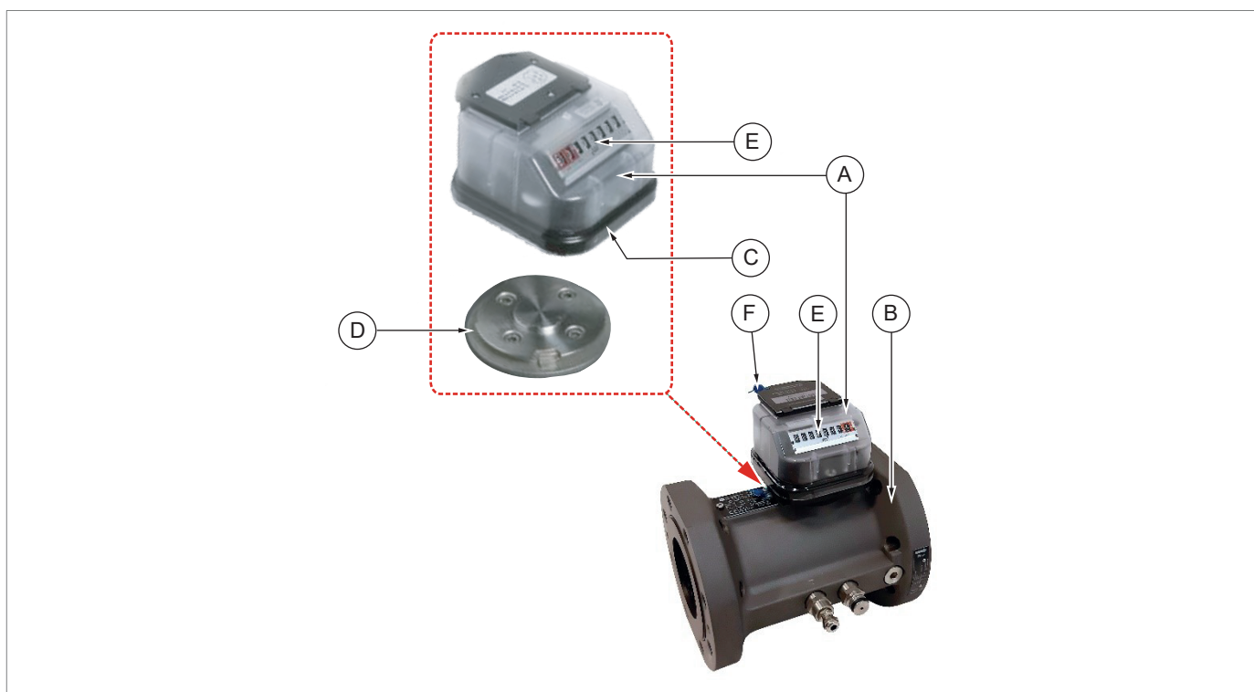
Fig. 4.4. Grupo totalizador
