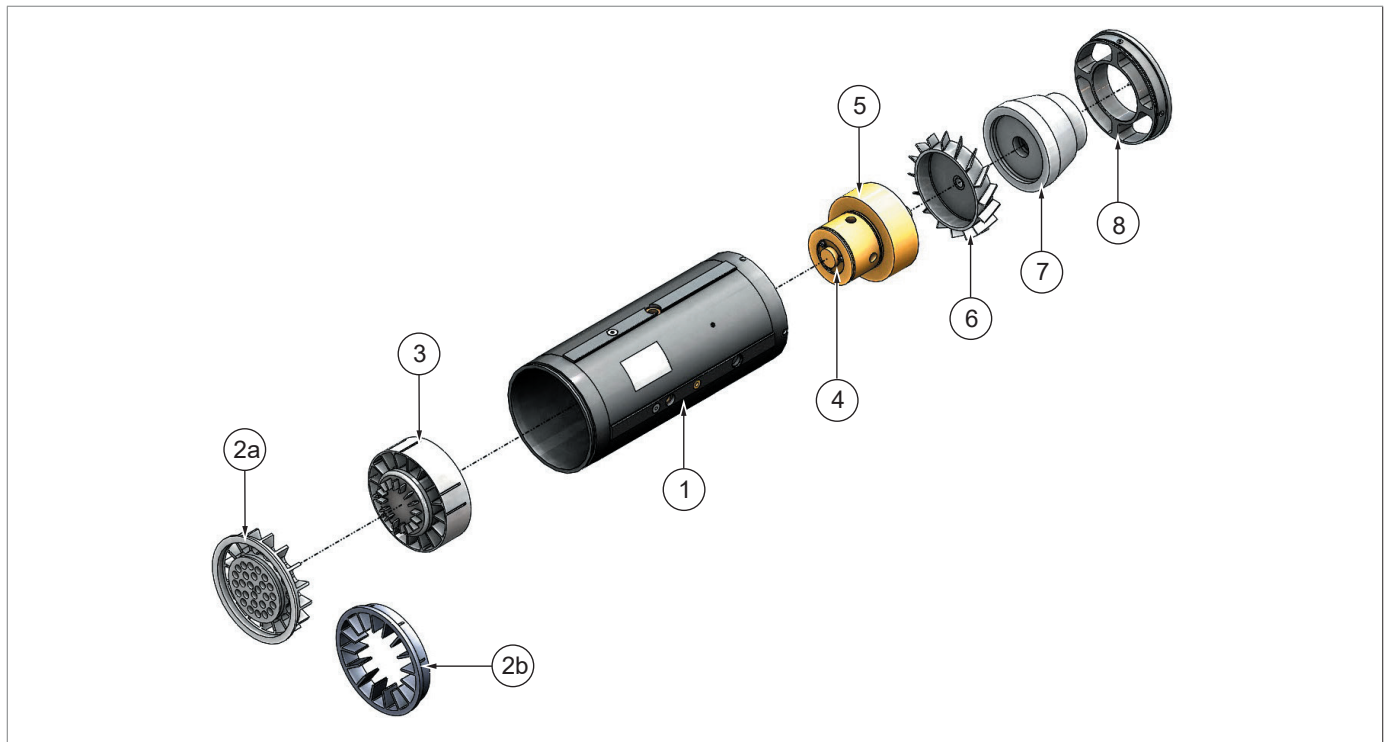
Fig. 4.3. Unidad de cartucho de medición
