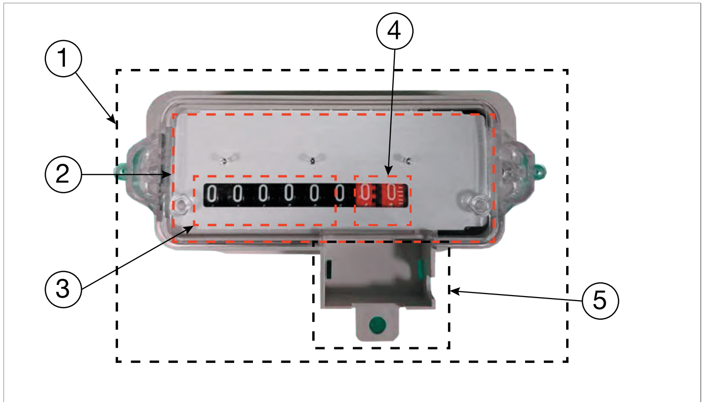
Fig. 5.3. Totaliser
