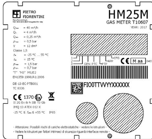
Fig.5 - Etichetta frontale HM25M -
