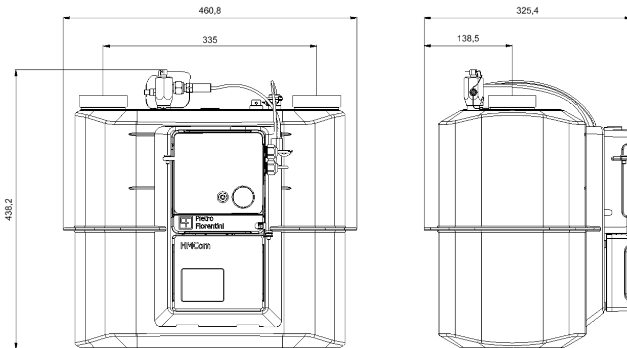
Fig.9 ingombri HM25M, attacco al processo 2"1/2 ISO 228-1
