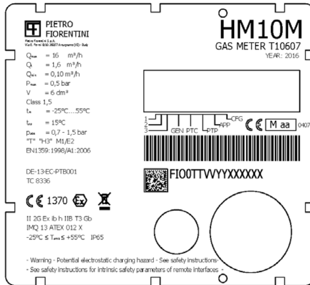
Fig.3 - Etichetta frontale HM10M -
