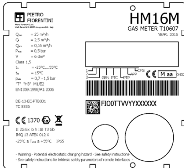
Fig.4 - Etichetta frontale HM16M -
