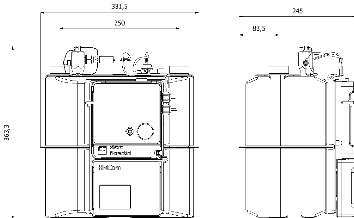
Fig.7 ingombri HM10M, attacco al processo 1"1/4 ISO 228-1
