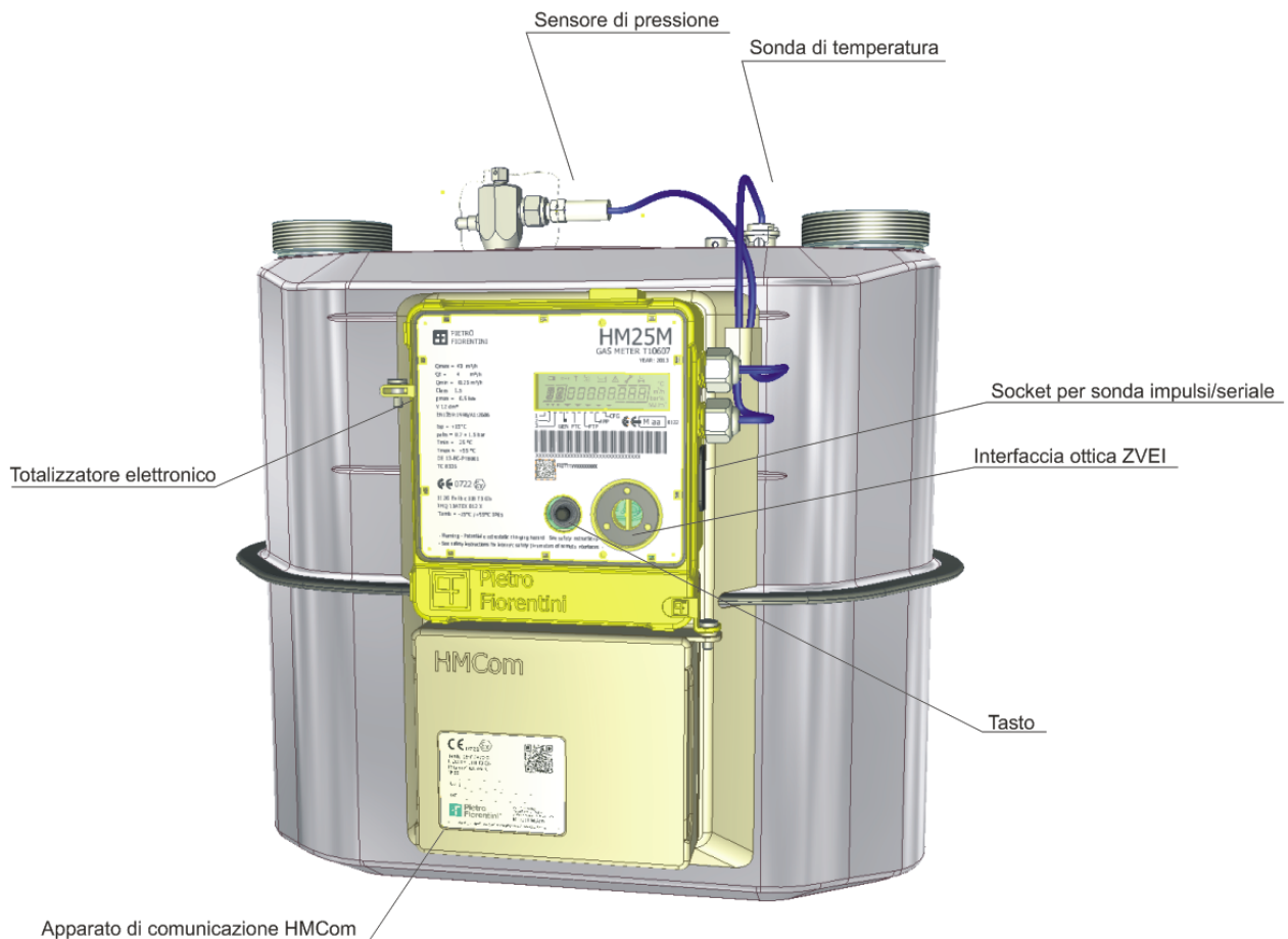
Fig.6 Overview HM25M ( l'immagine è rappresentativa di tutta la gamma ) -
