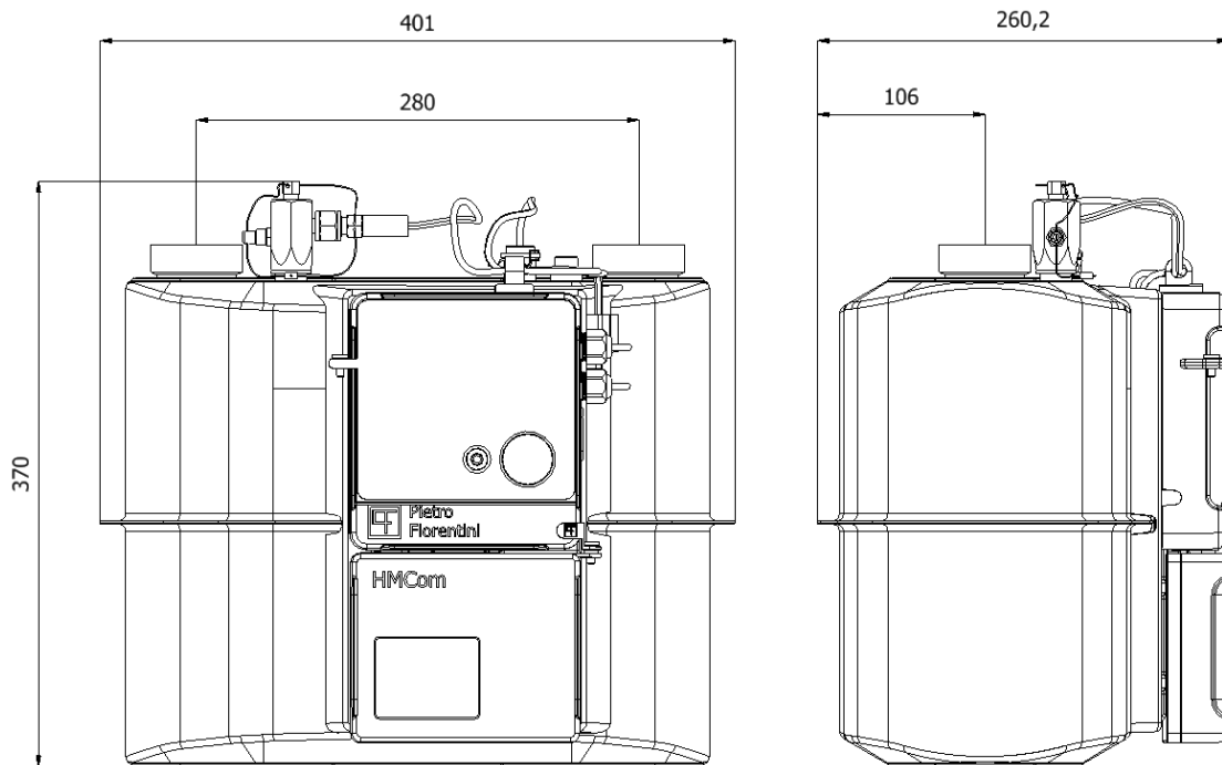
Fig.8 ingombri HM10M/16M, attacco al processo 2" ISO 228-1
