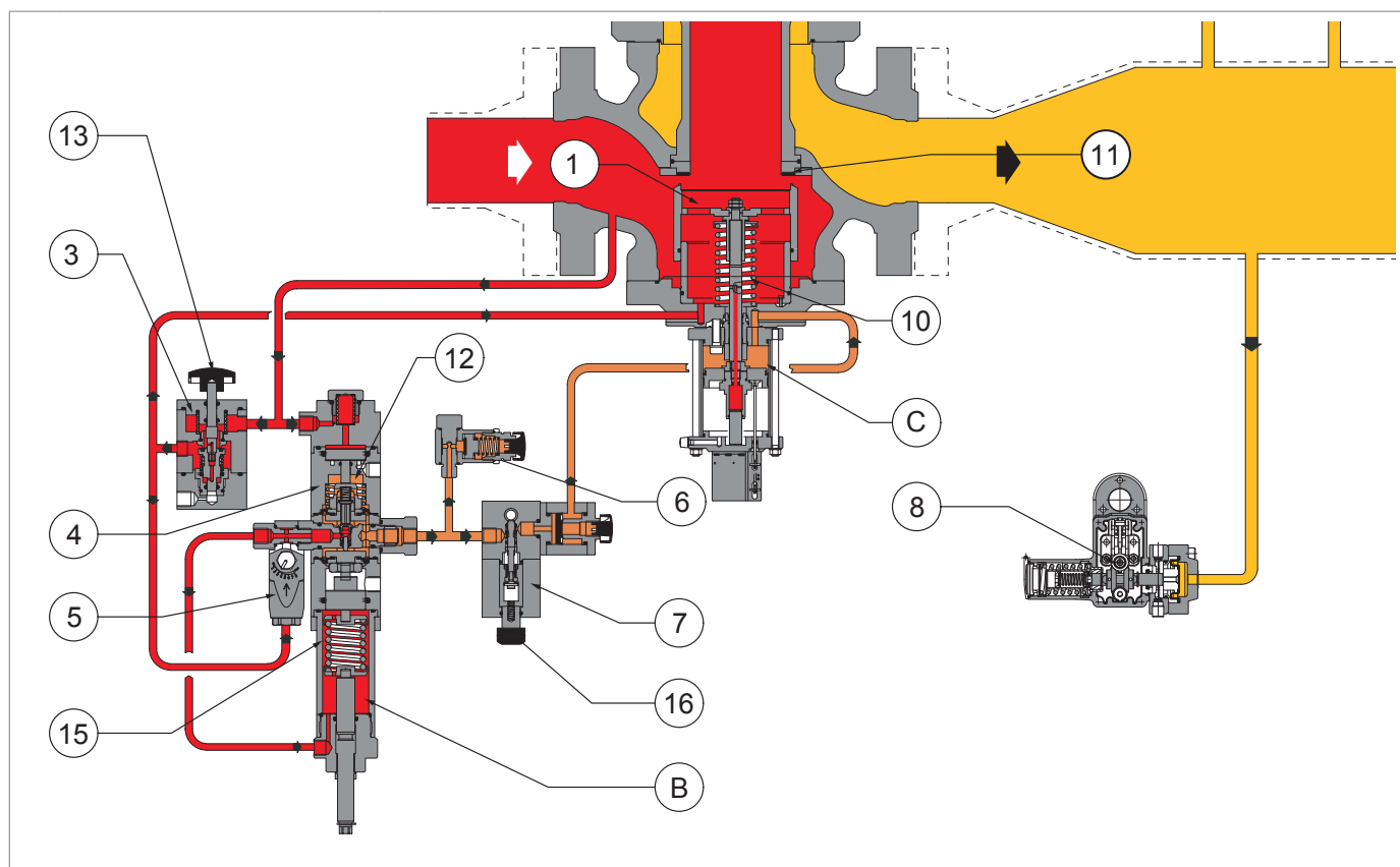
■ Ciśnienie przed urządzeniem ■ Ciśnienie za urządzeniem ■ Ciśnienie zasilania siłownika
