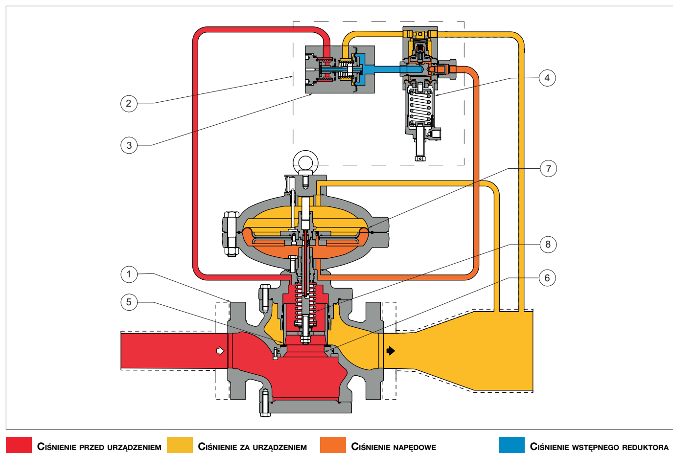
Rys. 4.1. Opis ogólny REFLUX 819
