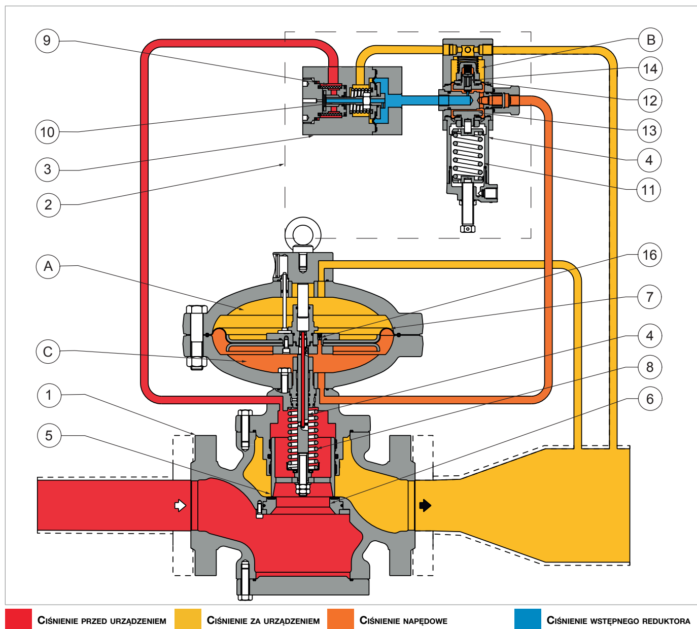
Rys. 4.2. Działanie REFLUX 819
