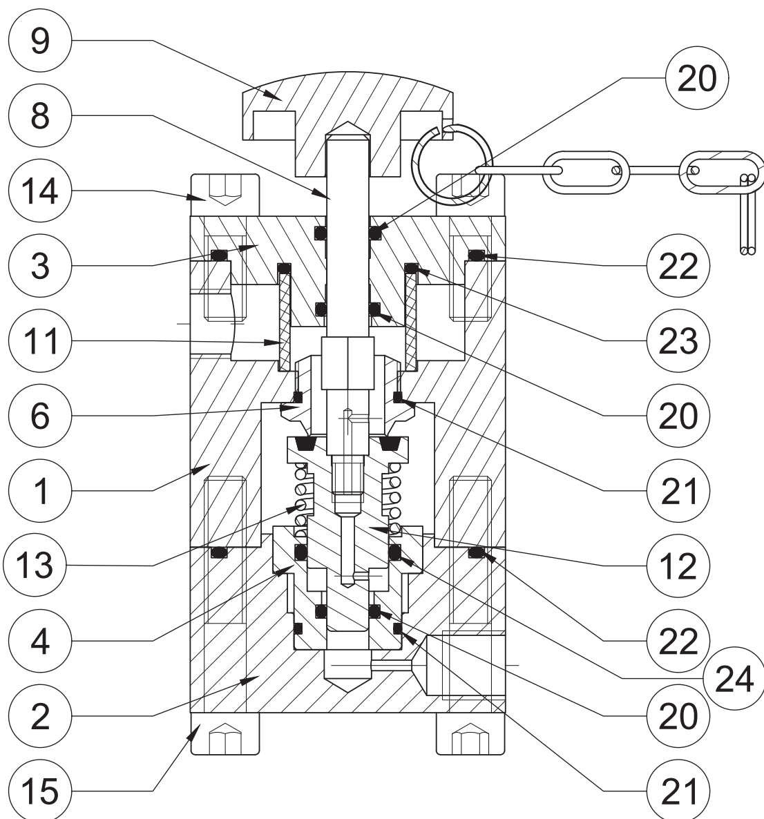
Urządzenie obciążeniowe HP2/2
