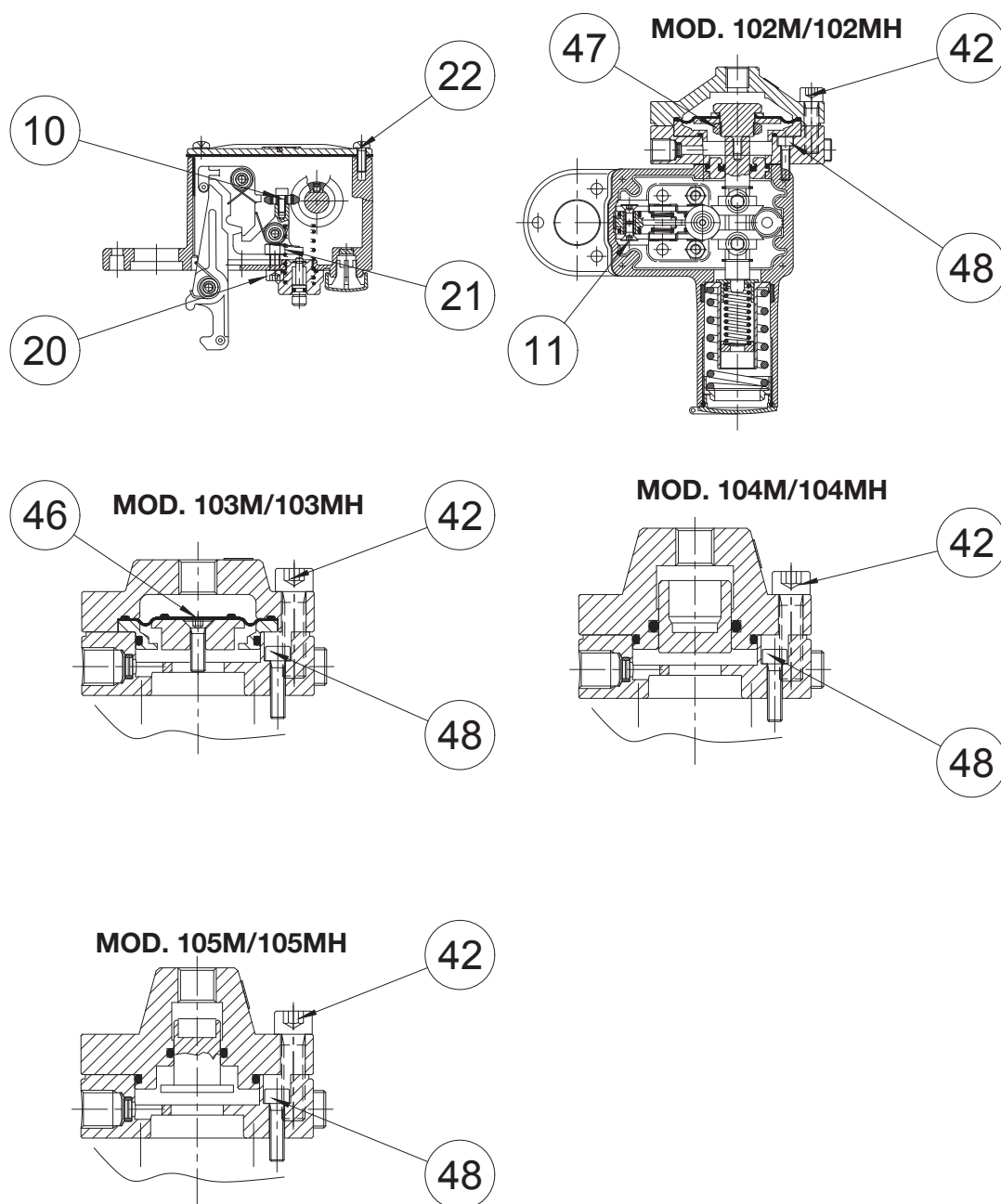
Rys. 9.49. Momenty dokręcania dla presostatów mod. 100
