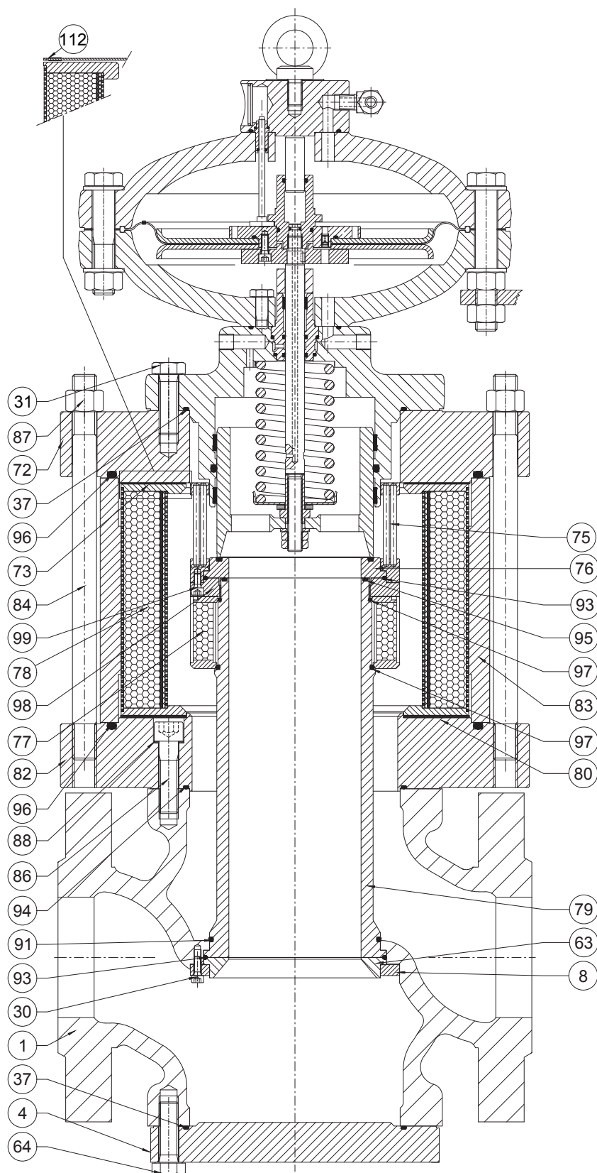
Tłumik DB/819
