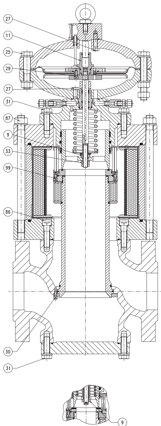
Rys. 9.40. Momenty dokręcania REFLUX 819 + Tłumik DB/819
