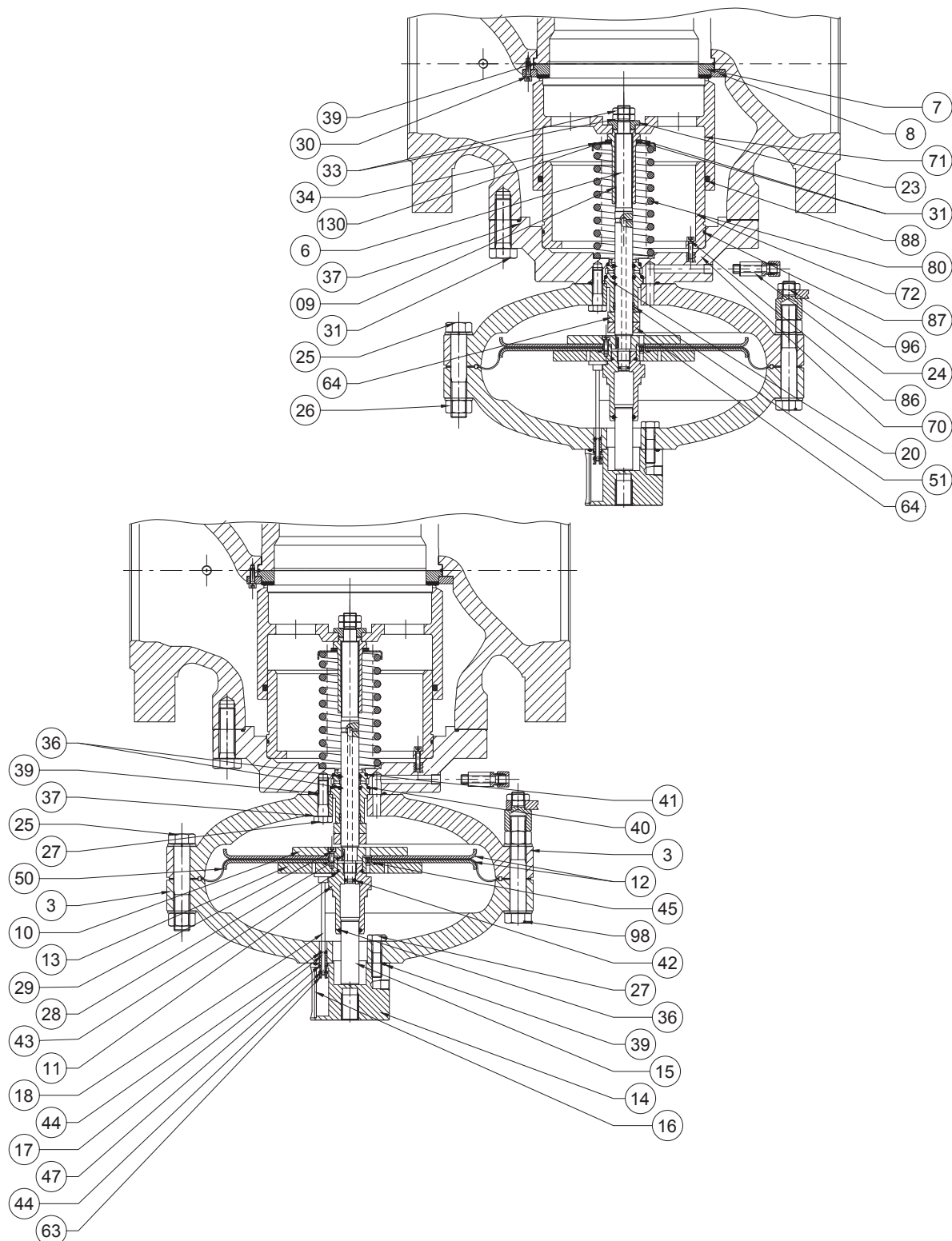
Wbudowany monitor PM/819 6"÷ 10"
