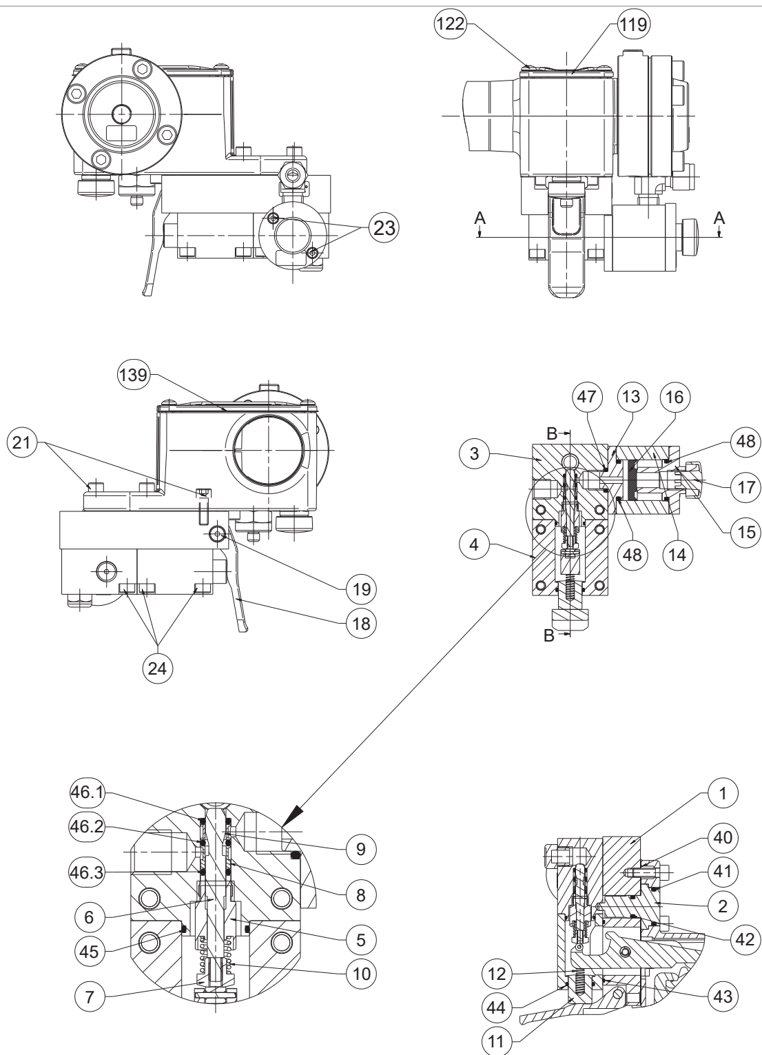
Rys. 9.83. Zawór 3/2
