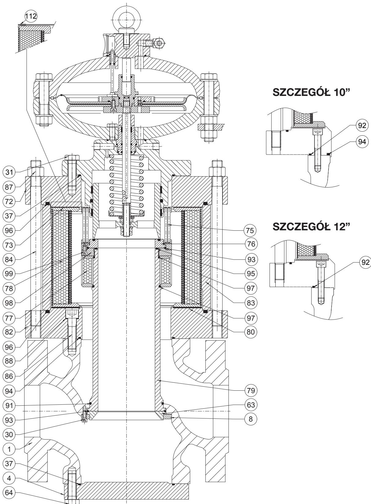
Rys. 9.60. Tłumik DB/819
