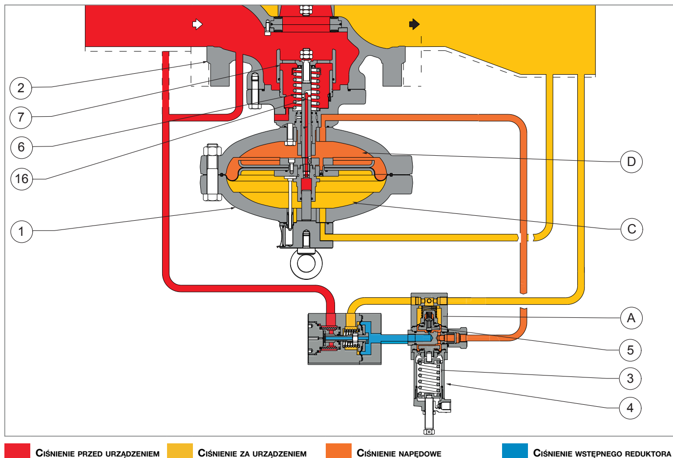
Rys. 4.8. Działanie wbudowanego monitora w przypadku awarii głównego regulatora
