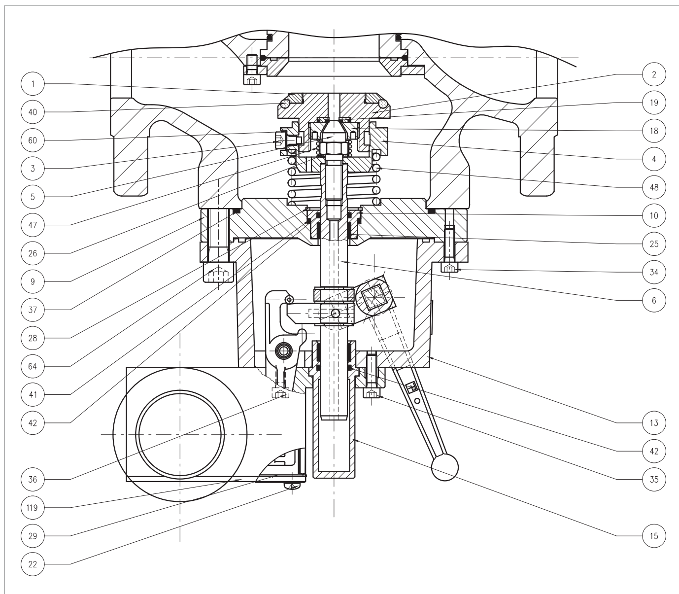
Rys. 9.71. Wbudowany zawór blokujący SB/82 2"÷ 3"
