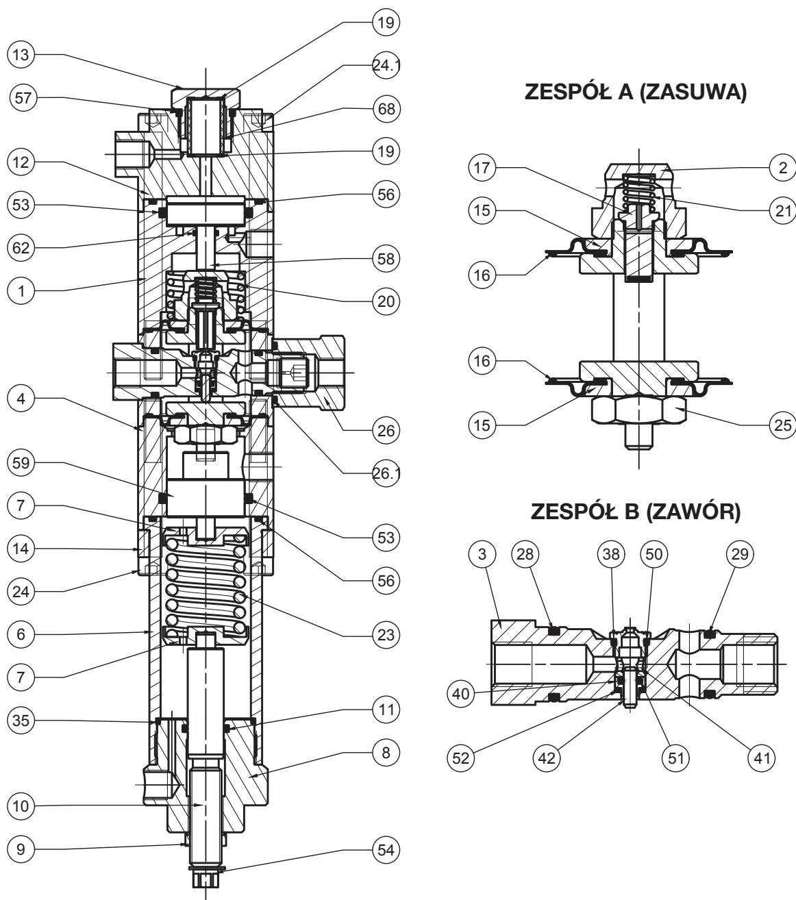
Rys. 9.81. Regulator ciśnienia R44/SS
