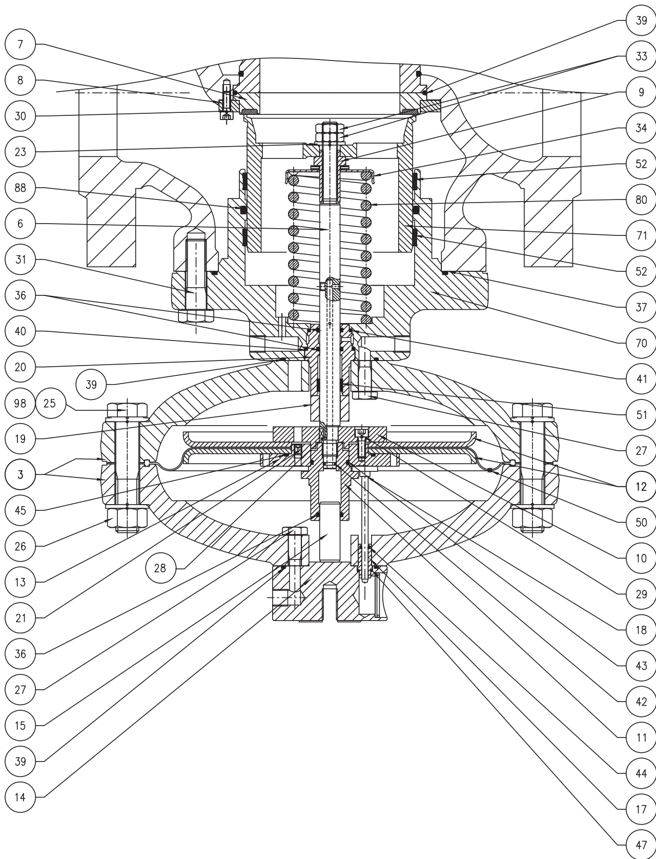
Wbudowany monitor PM/819 3"÷ 4"
