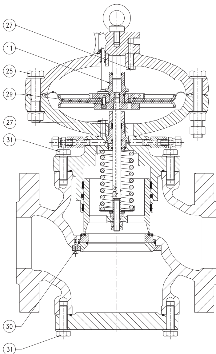
Momenty dokręcania REFLUX 819
