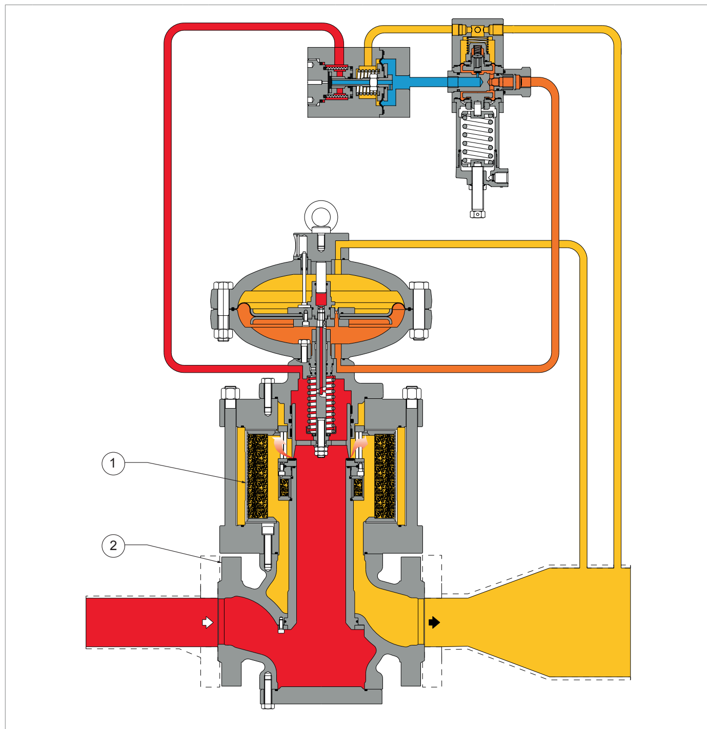
Rys. 4.3. Wbudowany tłumik DB/819
