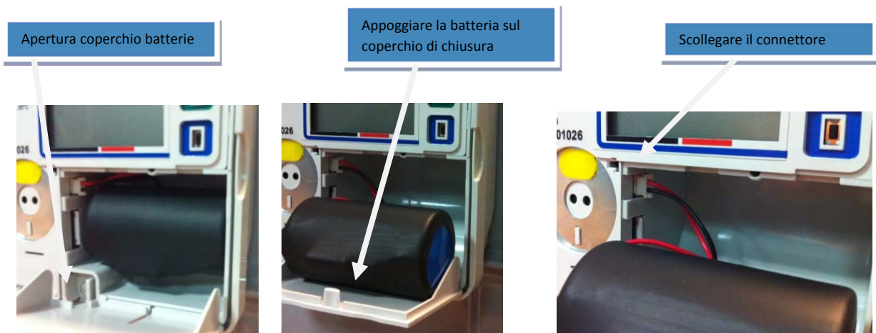
Figura 6 – Sostituzione batteria
