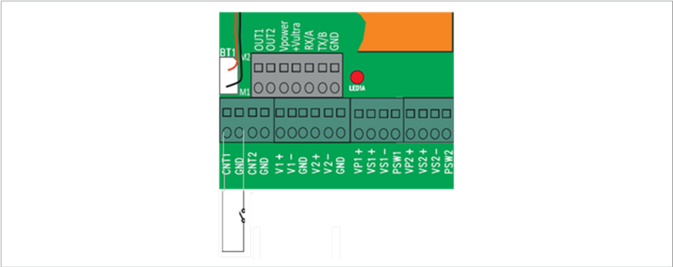
Fig. 4.5. Bloque de terminales de entradas digitales
