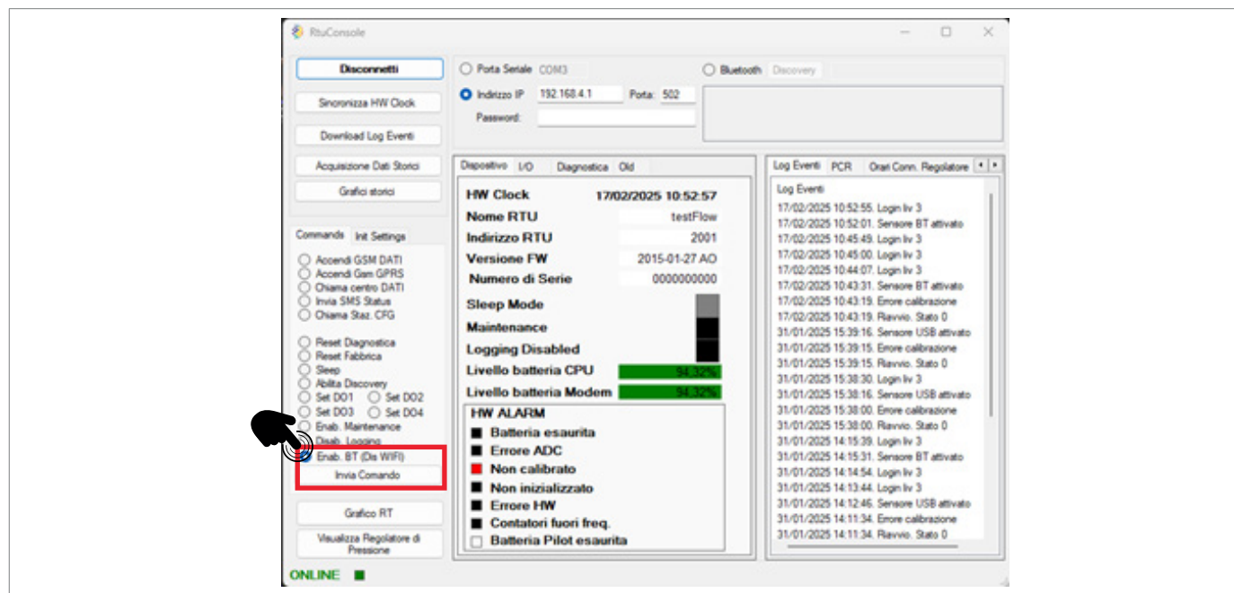
Fig. 5.14. Interfaz Rainbow para cambiar al modo Wi-Fi
