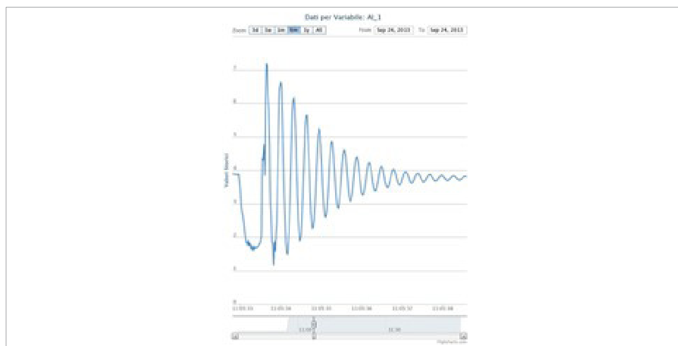
Fig. 8.37. Ejemplo de gráfico de muestreo
