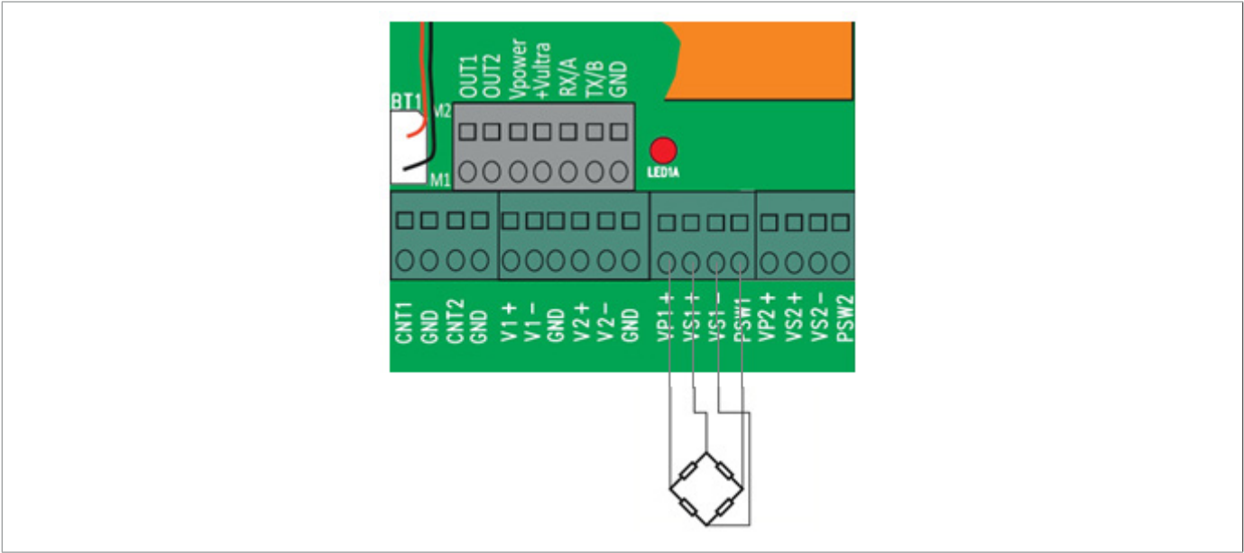
Fig. 4.4. Bloque de terminales de entradas de presión
