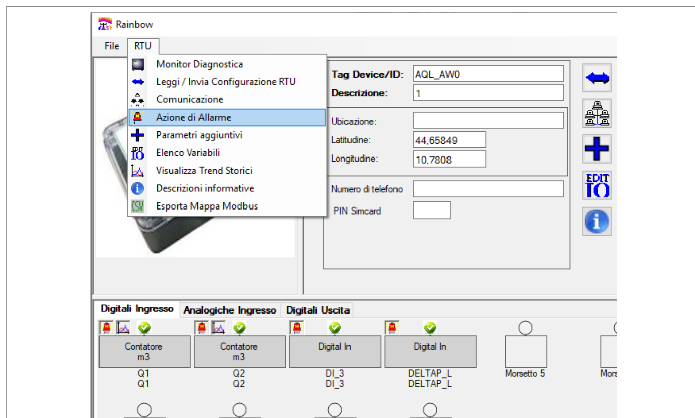
Fig. 8.48. Ventana de configuración de acciones de alarma
