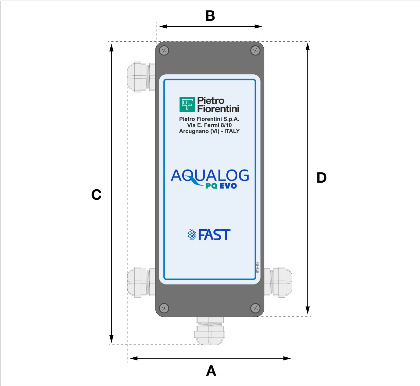
Fig. 6.15. Dimensiones AQUALOG PQ EVO vista frontal
