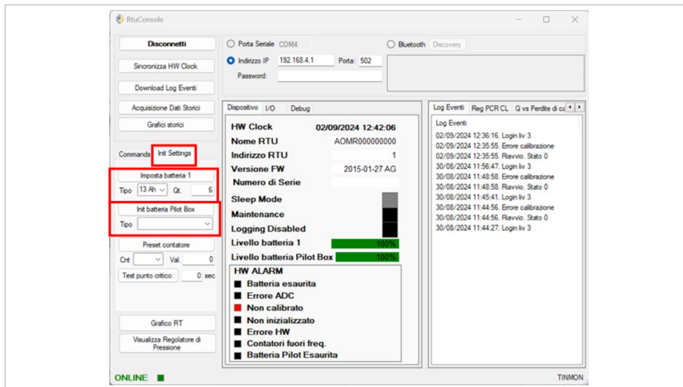
Fig. 8.47. Pantalla de inicialización de las baterías
