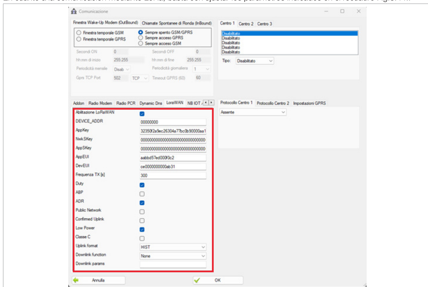
Fig. 8.44. Configuración de los parámetros de comunicación LoRa
