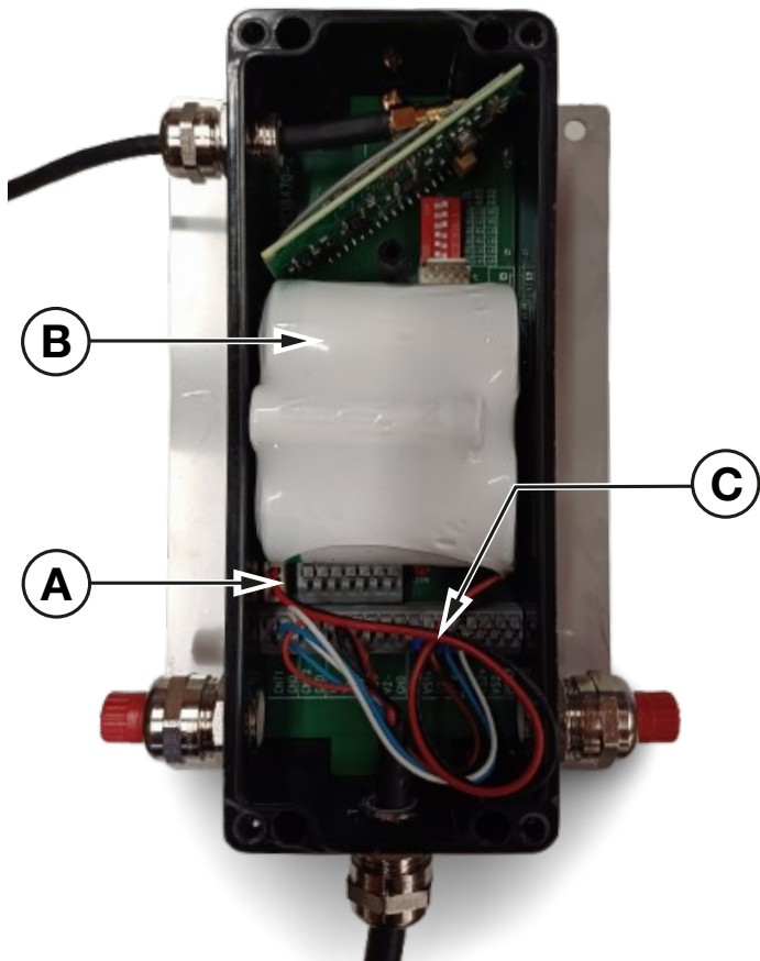
Fig. 9.56. Sustitución del paquete de baterías
