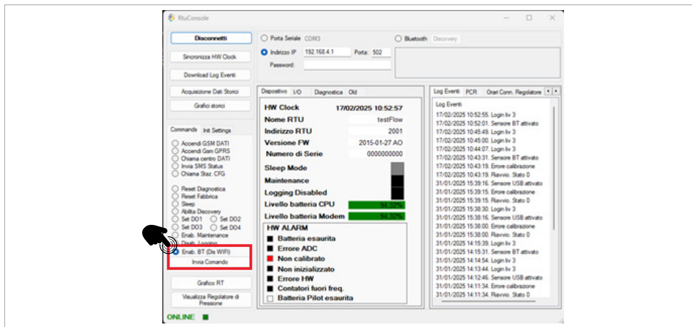
Fig. 5.12. Interfaz Rainbow para cambiar al modo Bluetooth
