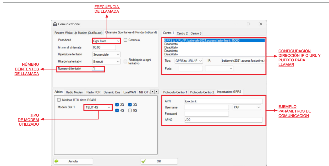
Fig. 8.42. Configuración de los parámetros de conexión para RTU con llamada 2G/ 3G/ 4G
