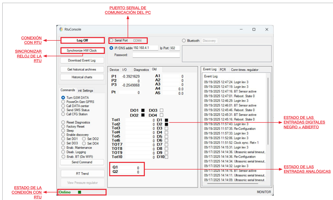
Fig. 8.46. Ventana de comunicación local con RTU
